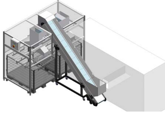
Pnömatik Kaydırma Konveyörü ve Çift Taraflı 3 Yollu Anahtarlar ile 12 Katlı Torba Dolum
