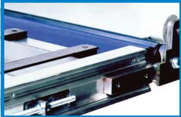
Konveyörün gövdesine entegre edilmiş kayış gerdirmeye mekanizması (kam sürgüsü), tüm açı aralığında sabit gerilim sağlar (patentli)
