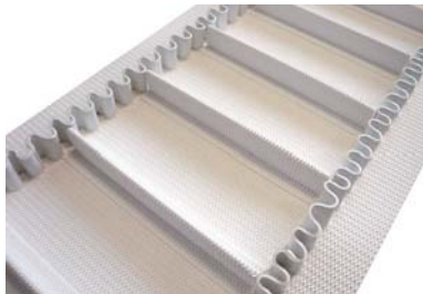
Fırırlı Kenar Bariyer Bant ve Bant Profili İçeren Örnek Bant
